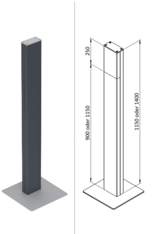
Variante mit großer Bodenplatte / Variant with large base plate
