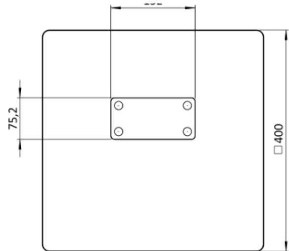
Variante mit großer Bodenplatte / Variant with large base plate
