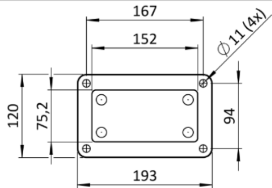
Variante mit großer Bodenplatte / Variant with large base plate
